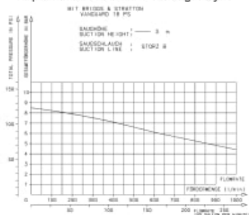
Kapasitetskurve Otter - 3m sugehøyde
